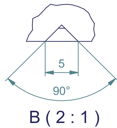
RAINURE OPTIONNELLE
