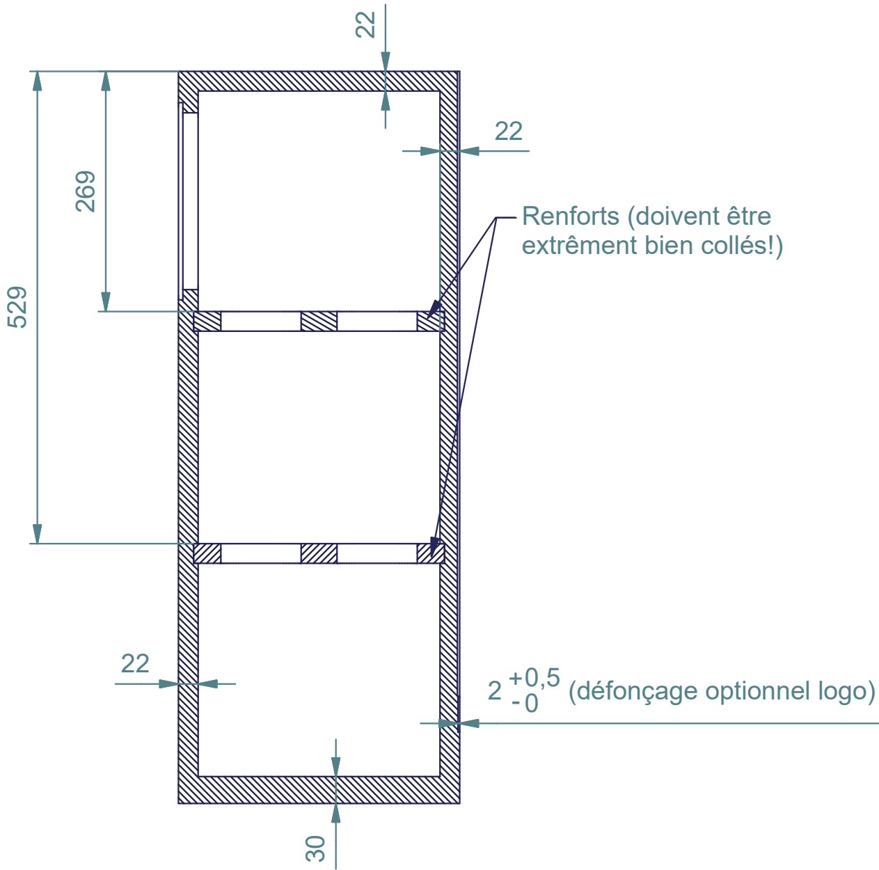
A-A ( 0,12 : 1 )
